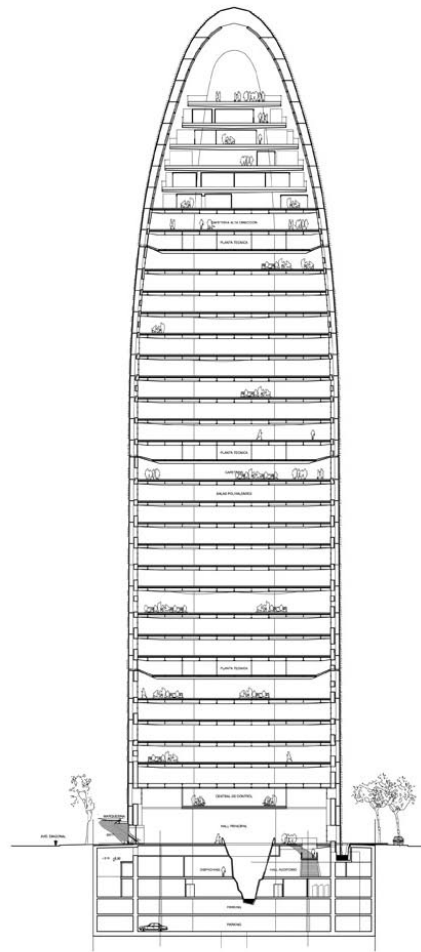
SECCION NORTE - SUR
