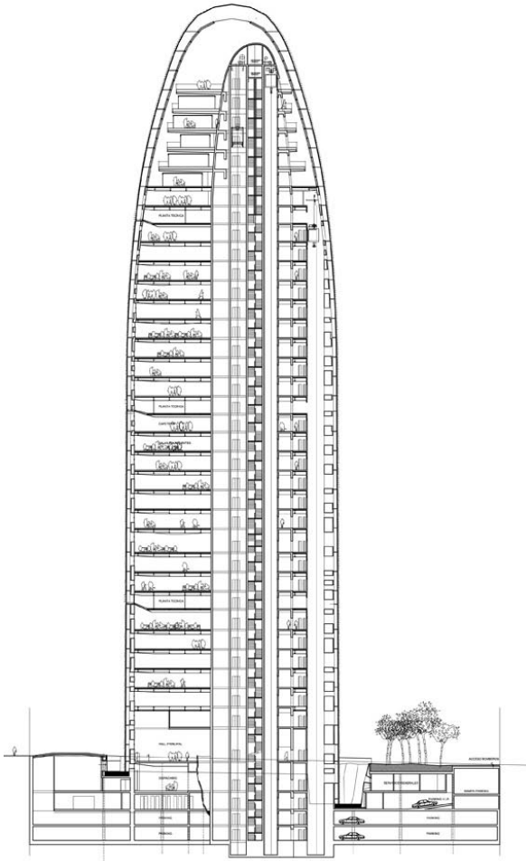
SECCION OESTE - ESTE
