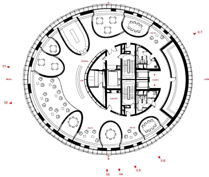
PLANTA 25. CAFETERÍA ALTA DIRECCIÓN.
